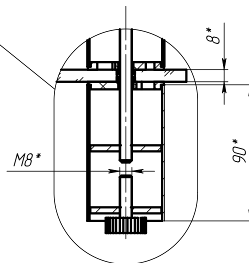
Угловая тумба Rescorner 750x450 № 12132 Каркас: Серебристый муар. Стекло: Прозрачное.
